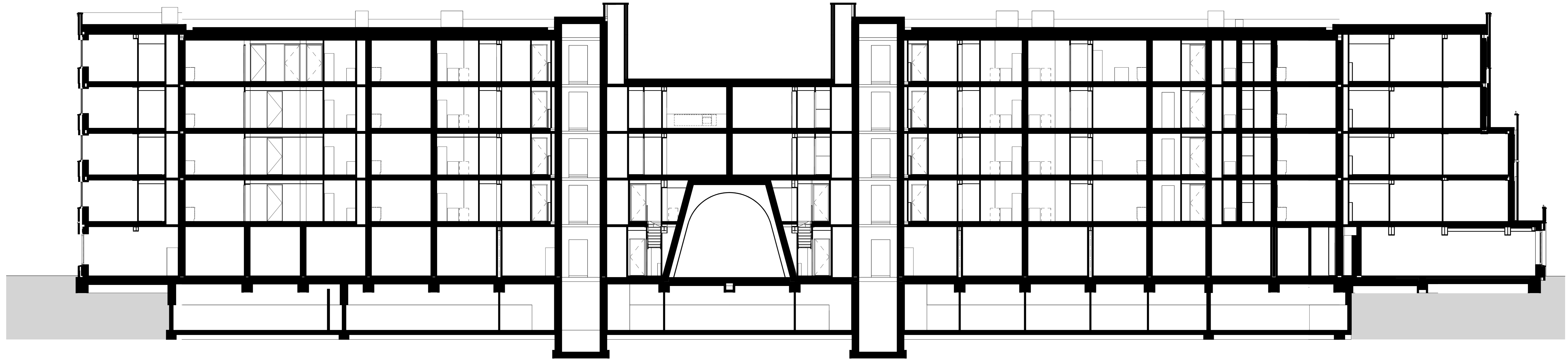
Doorsnede AA
