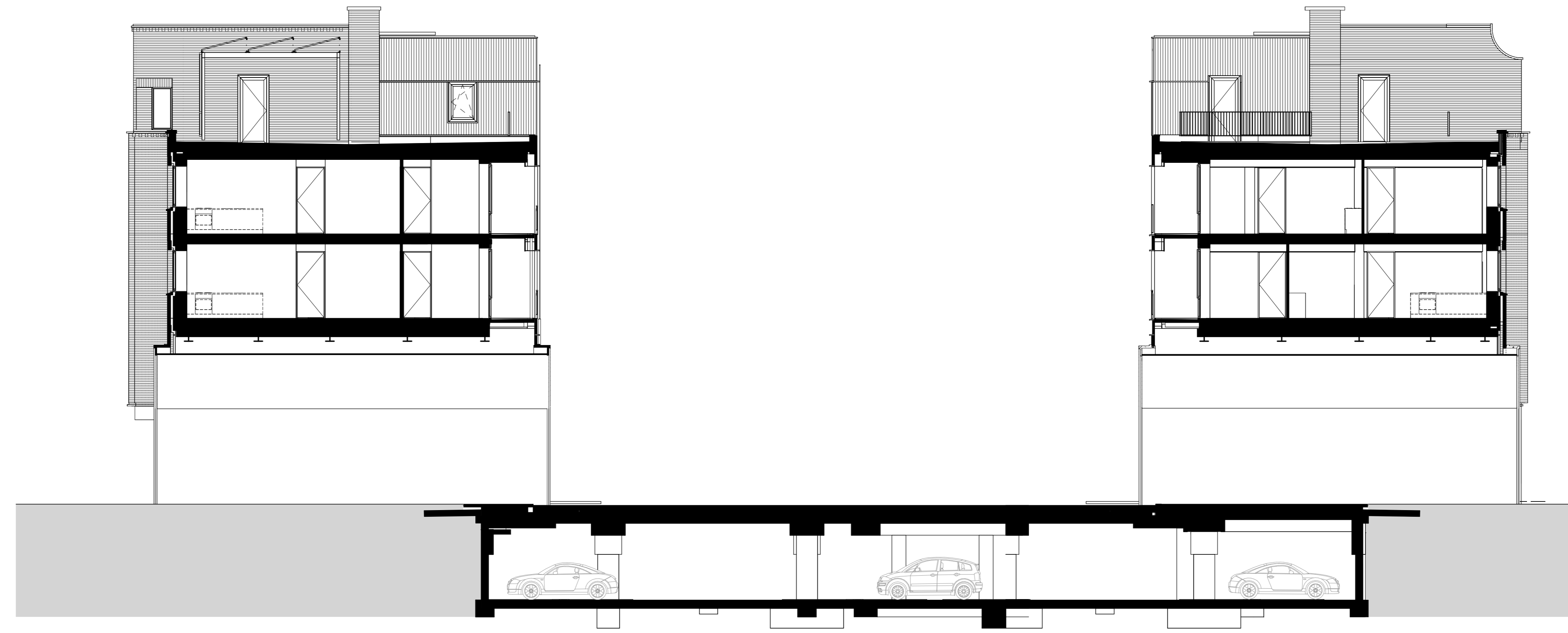
Doorsnede CC
