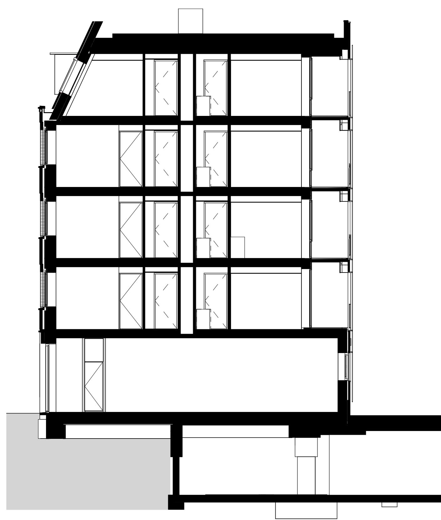
Doorsnede BB
